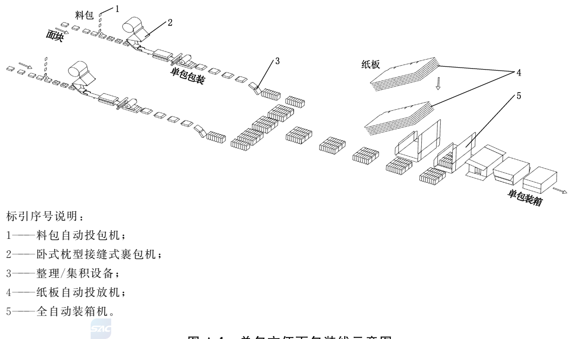
图 A.1 单包方便面包装线示意图
